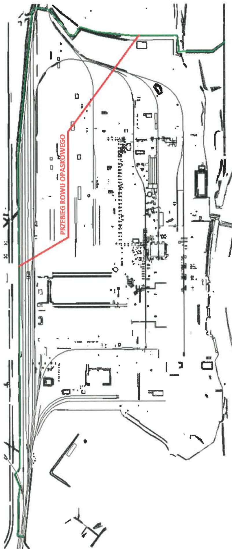
Rys. 2. Przebieg rowu opaskowego elektrowni
